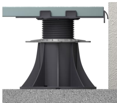
Profil PEDall DISTANCE PP s dlažbou
