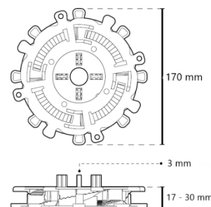
Rozměry PEDall CLASSIQ 17-30mm
